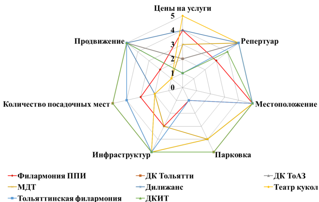
Рисунок 5 – Многоугольник конкурентоспособности
